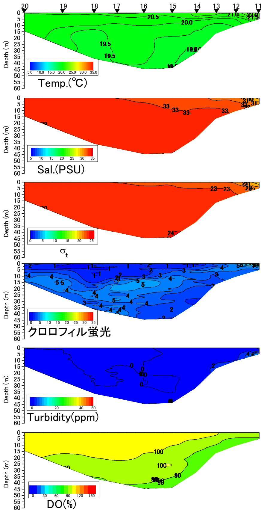
八代海中央ラインの水温(°C)、塩分、密度( \sigma_t )、クロロフィル蛍光強度、濁度、溶存酸素飽和度(DO%)の鉛直面図(国土交通省の調査による) (2014年5月30日)
